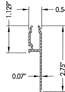
17 SILL RISER 356-A51-A
